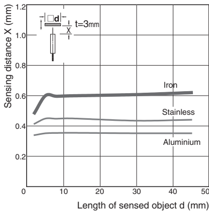
E2C-EM07(-□)
