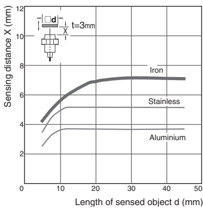
E2C-EM07(-□)
